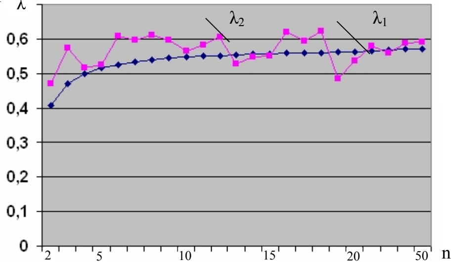
Рис. 1 – Зависимость величины \lambda_1 и \lambda_2 от объема выборки n
