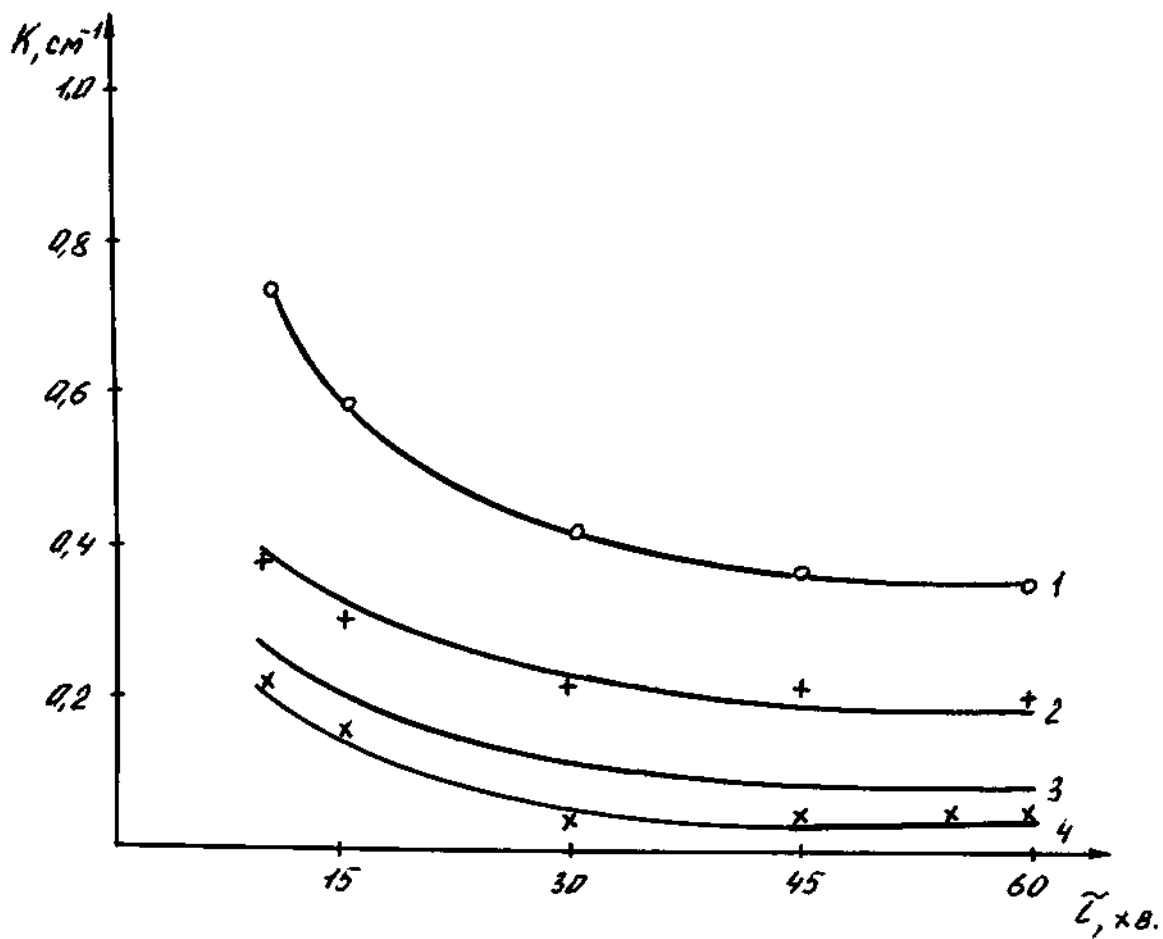
Рис. 1. Відстій завислих речовин у воді, скоагульованих 0,005%-ним розчином полімерів: 1 – без коагулянту; 2 – МАТАС; 3 – КОМЕТА; 4 – сополімер акриламід з ГДАХ
