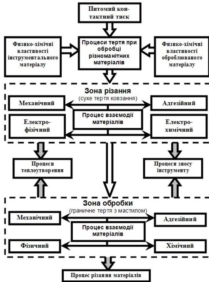
Рис. 1 – Існуюча фізична модель процесу тертя при обробці різноманітних матеріалів: світлими стрілками показаний напрям первинної взаємодії; темними - вторинного; тонкими чорними – внутрішня взаємодія між фізичними явищами процесу тертя
