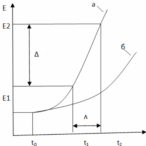
Рис. 1 – Залежність енерговитрат від величини знімаємого шару: а – для ідеальних кристалів; б – для реальних металів.
