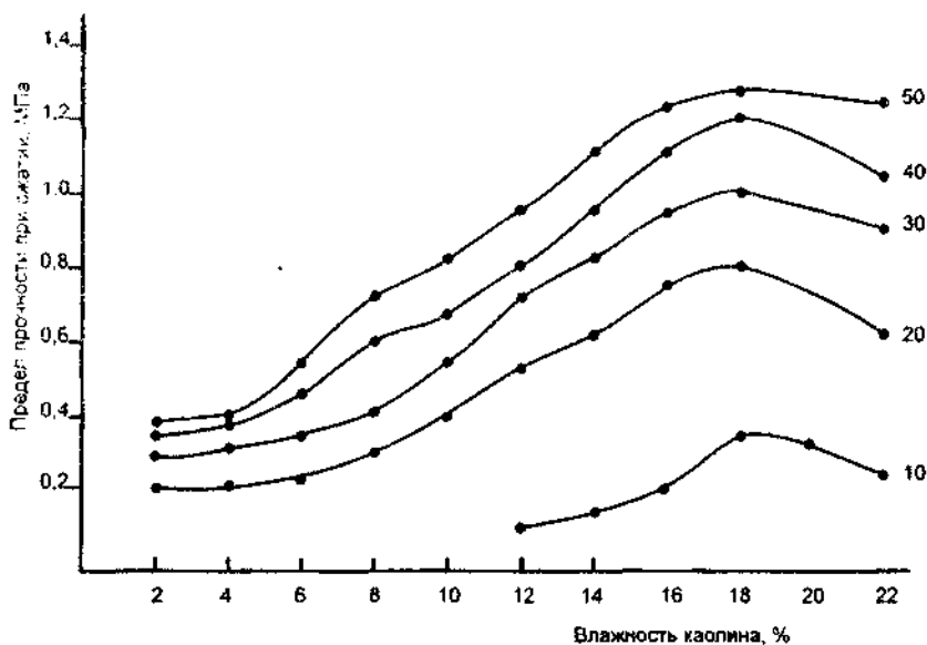
Рис. 3. Зависимость предела прочности при сжатии брикетов от влажности каолина (цифры на кривых – величина давления прессования, МПа)
