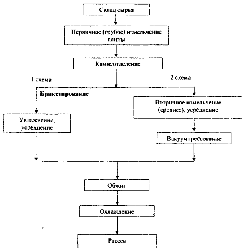
Рис. 1. Технологическая схема производства шамота
